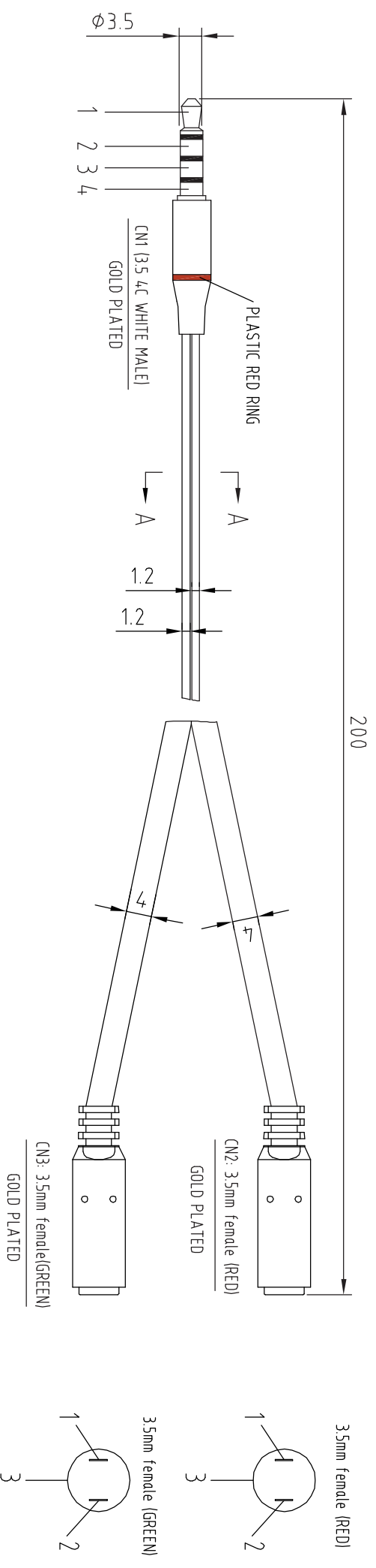
SCALE 10:1 A:A
